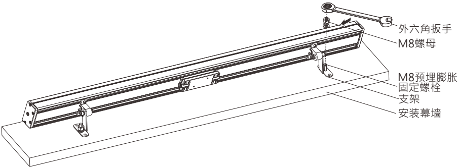
用螺丝将灯具支架与安装幕墙固定
