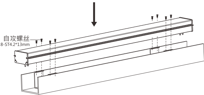
灯具安装孔对齐支架安装孔，用螺丝锁紧
