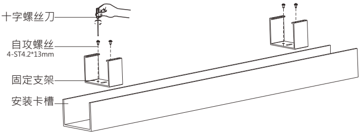
用螺丝将灯具支架与安装卡槽固定
