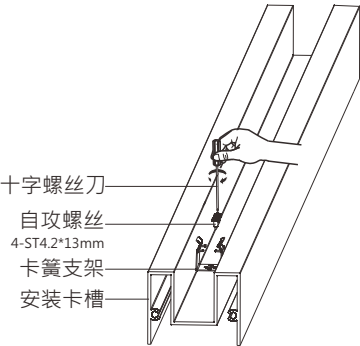
用螺丝将灯具支架与安装卡槽固定
