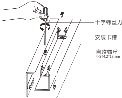
用螺丝将灯具支架与安装卡槽固定
