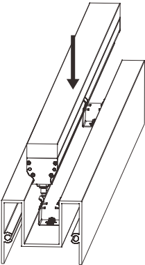
灯具卡进支架
