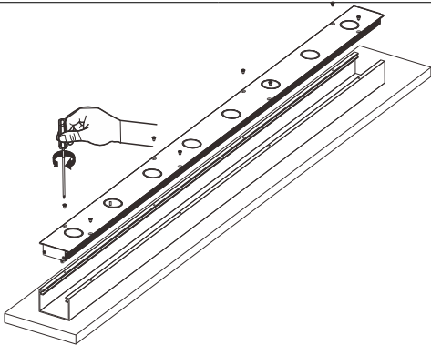
灯具飞翼安装孔对齐安装卡槽螺丝孔，用螺丝固定
