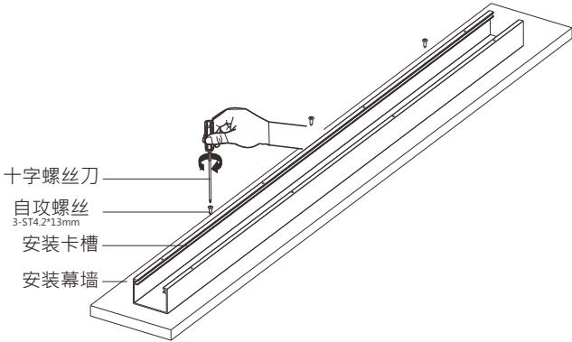
用螺丝将安装卡槽与安装幕墙固定
