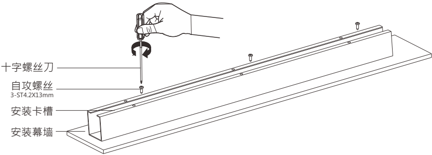
用螺丝将安装卡槽与安装幕墙固定
