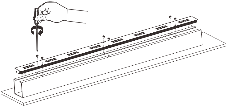
灯具飞翼安装孔对齐安装卡槽螺丝孔，用螺丝固定
