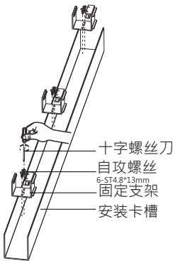
用螺丝将灯具支架与安装卡槽固定
