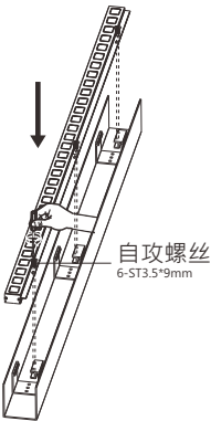
灯具飞翼安装孔对齐支架螺丝孔，用螺丝固定
