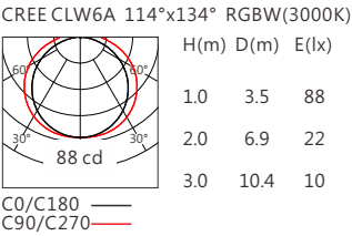
RGBW(3000K) 352 lm
