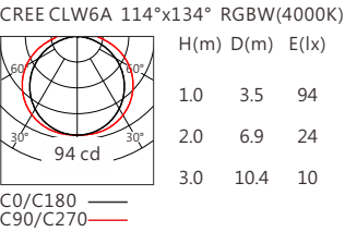
RGBW(4000K) 375 lm
