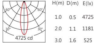
3535 30° RGBW(4000K)
