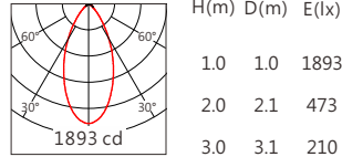
3535 55° RGBW(4000K)
