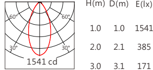
3535 55° RGBW(3000K)
