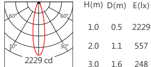
3535 30° RGBW(3000K)
