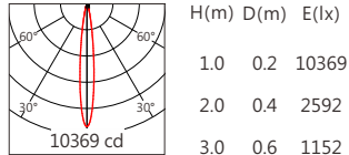
3535 12° RGBW(4000K)
