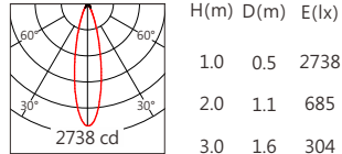
3535 30° RGBW(4000K)
