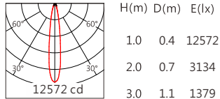
CMU1013 15° 3000K
