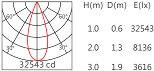
Bridgelux BXKC 36° 4000K
