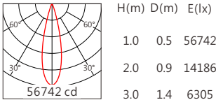
Bridgelux BXKC 24° 4000K
