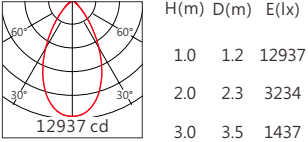
Bridgelux BXKC 60° 4000K
