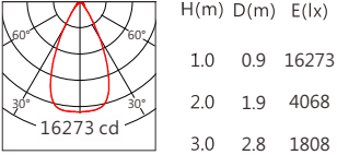
Bridgelux BXKC 50° 4000K
