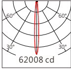
5050 9° RGBW(4000K)
