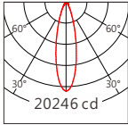
5050 30° RGBW(3000K)
