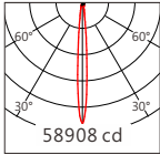
5050 9° RGBW(3000K)
