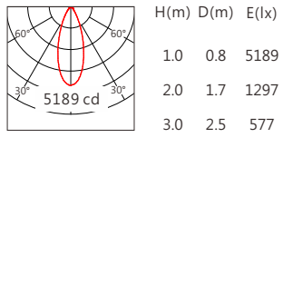
CREE XP-L HIC 45° RGBW(3000K)
