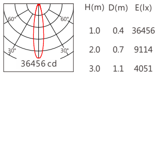
CREE XP-L HIC 20° RGBW(3000K)
