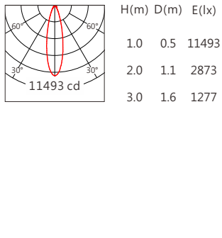
CREE XP-L HIC 30° RGBW(3000K)
