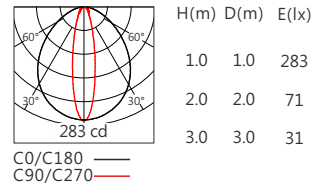
CREE CLW6A 20°x90° RGBW(3000K)
