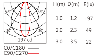
CREE CLW6A 35°x90° RGBW(3000K)
