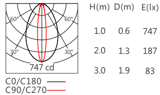
CREE CLW6A 16°x60° RGBW(4000K)
