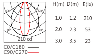
CREE CLW6A 35°x90° RGBW(4000K)
