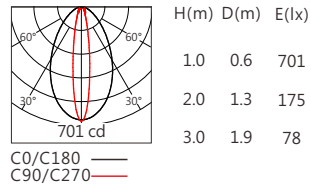
CREE CLW6A 16°x60° RGBW(3000K)
