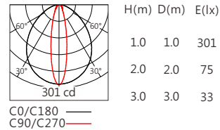
CREE CLW6A 20°x90° RGBW(4000K)
