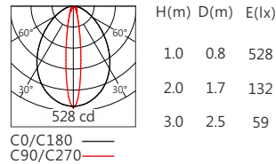
CREE CLW6A 16°x80° RGBW(3000K)
