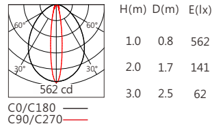
CREE CLW6A 16°x80° RGBW(4000K)
