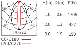
OSRAM 2835 12°x60° 2700K+6500K
