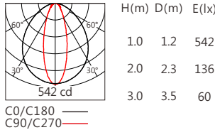
OSRAM 2835 30°x90° 3000K+5000K
