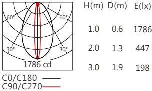
OSRAM 2835 12°x60° 3000K+5000K
