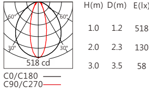
OSRAM 2835 30°x90° 2700K+6500K
