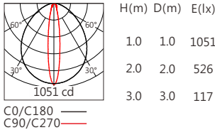
OSRAM 2835 16°x90° 3000K+5000K
