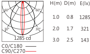
OSRAM 2835 12°x80° 2700K+6500K
