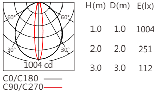
OSRAM 2835 16°x90° 2700K+6500K
