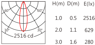
5050 30° RGBW(3000K)
