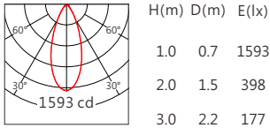
5050 40° RGBW(3000K)
