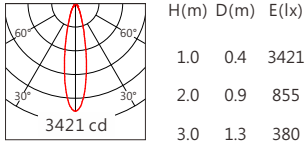
5050 25° RGBW(4000K)
