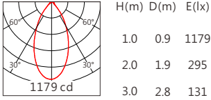
5050 50° RGBW(4000K)
