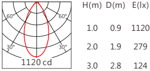
5050 50° RGBW(3000K)
