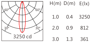
5050 25° RGBW(3000K)
