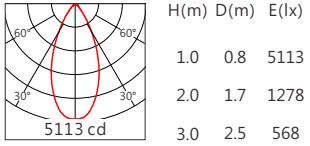
OSRAM SSL80 45° 4000K
