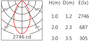
OSRAM SSL80 60° 4000K
