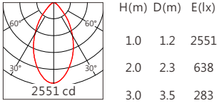
OSRAM SSL80 60° 3000K
