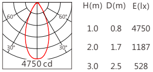
OSRAM SSL80 45° 3000K
