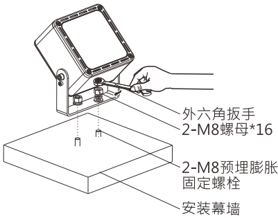
用螺丝将灯具支架与安装幕墙固定
