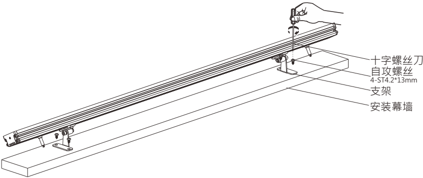
用螺丝将灯具支架与安装幕墙固定
