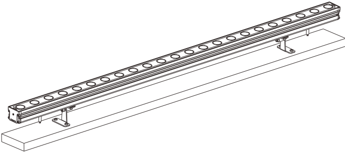
将灯具旋转到合适的角度，安装完成
